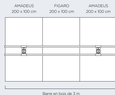
Barre en bois de 3 m
