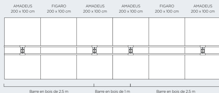
Barre en bois de 2,5 m Barre en bois de 1 m Barre en bois de 2,5 m
